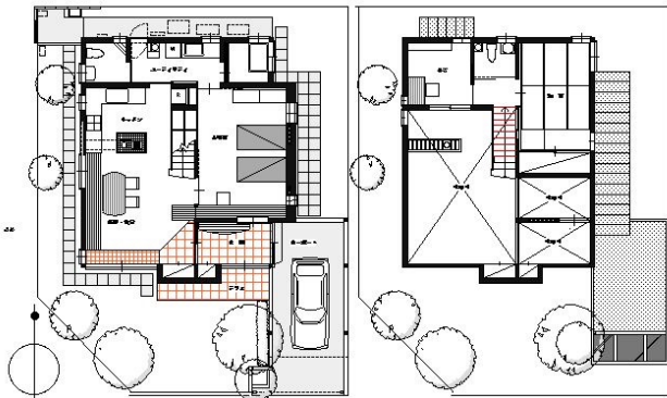
吉井町の家 1階平面図
