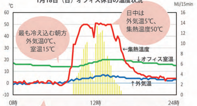
1月18日（日）オフィス休日の温度状況
